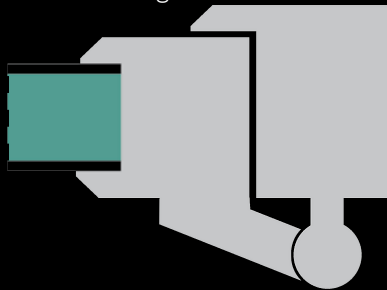
Aufsatz-Füllung einseitig flügelüberdeckend
